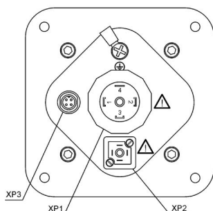
ТКП-100/М2. Вид сзади. Разъемы GSP 311 (XP1), GSSNA 300 (XP2), М-614А-ВNGD (XP3)
