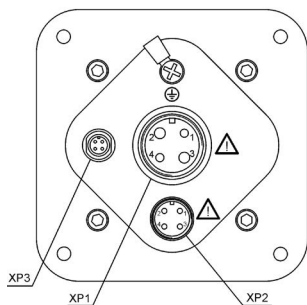
ТКП-100/М1. Вид сзади. Разъемы 2РМ 22 (XP1), 2РМ14 (XP2), М-614А-ВNGD (XP3)
