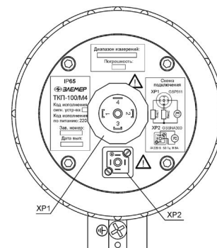
ТКП-100/М4. Вид сзади. Разъемы GSP 311 (XP1), GSSNA 300 (XP2)
