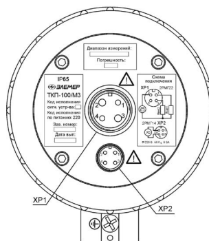
ТКП-100/М3. Вид сзади. Разъемы 2РМ 22 (XP1), 2РМ14 (XP2)
