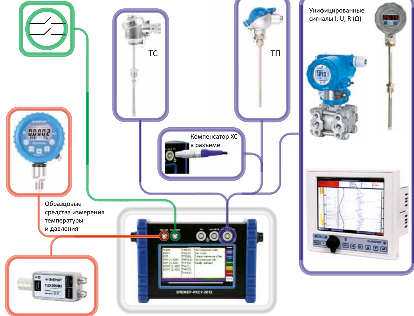
Тестирование реле 2 канала
