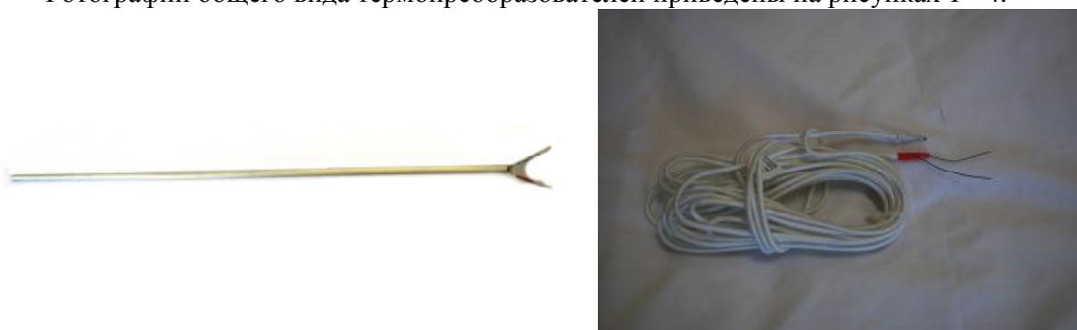
Рисунок 1 - Общий вид бескорпусных ДТП модификации ХХ1
