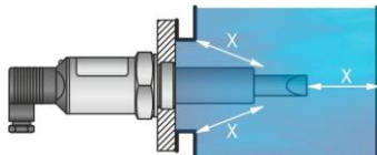
Модель с фланцем, предельное расстояние x > 5 мм
